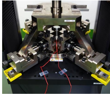
二軸引張試験用治具
